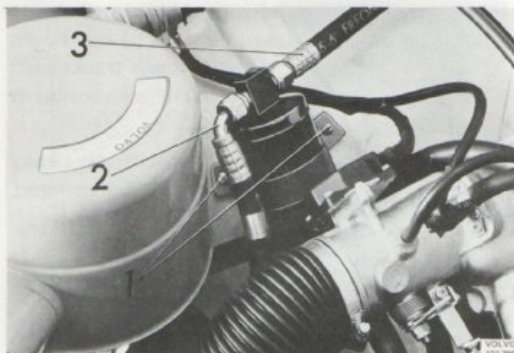
Bild 72. Torkare 140
