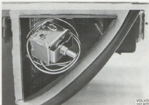
Bild 84. Placering av termostat i förångaraggregatets öppning
