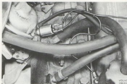
Bild 80. Magnetventil monterad i Stromberg förgasare
