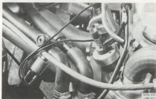
Bild 83. Magnetventil monterad på B 30 E motor
