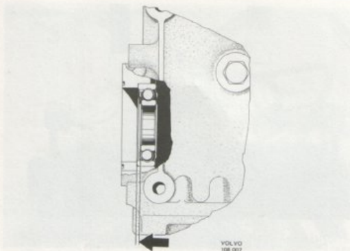
Bild 64. Montering av främre vevaxellager (A 206)
