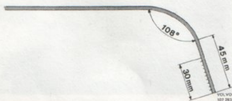
Bild 46. Oljesticka för kompressor
