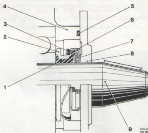
Bild 48. Vevaxeltätning
