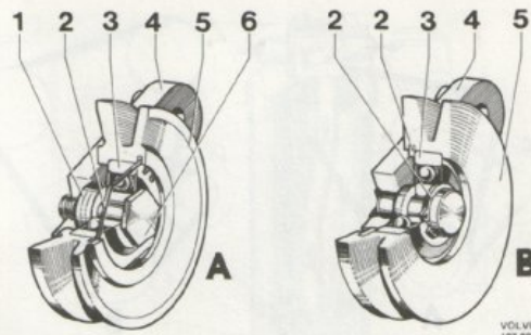
Bild 16. Spännrullar
