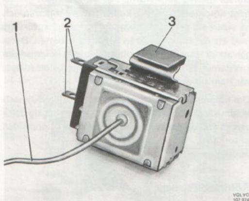
Bild 24. Termostat sen.utf.
