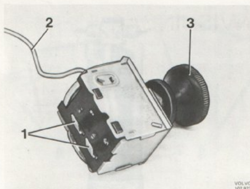
Bild 23. Termostat tid.utf.
