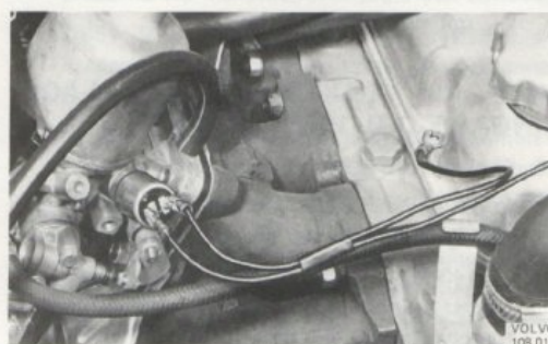
Bild 81. Magnetventil monterad i SU-förgasare
