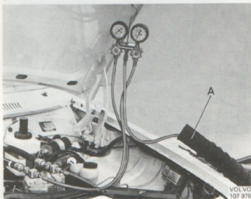
Bild 26. Tömning av köldmedium A. Avgasutslutnings slang
