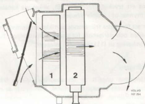
Bild 11. Luftströmningen genom centralenheten 1. Förångare 2. Värmecellpaket
