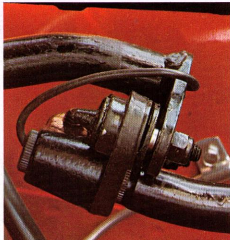
Delad rattstång av säkerhetstyp.
