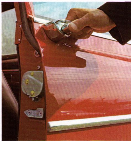
Krocksäkra dörrlås.
