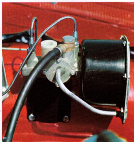
Bromsservo för snabbare, säkrare inbromsningar.
